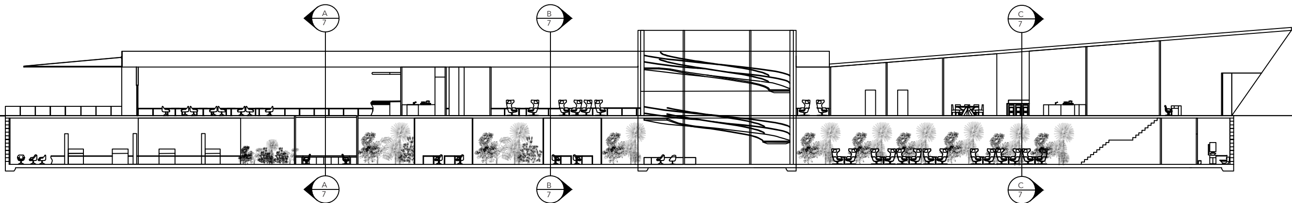
SECTION SCALE: 1:300
